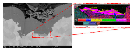
Coupe transversale de l'interface acier-dépôt de corrosion formé à 80 °C, sous 0,54 bar de \text{CO}_2 , à pH=6,6 au bout de 12 jours. Les différentes phases ont été détectées par analyse MEB-EBSD.
