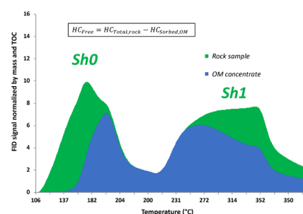
Principe de la nouvelle méthodologie de quantification des hydrocarbures liquides libres.
