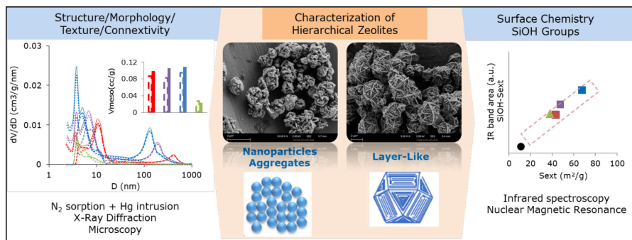
Caractérisation morphologique, texturale et de surface de différentes zéolithes à porosité hiérarchisée utilisées pour la séparation des xylènes.
